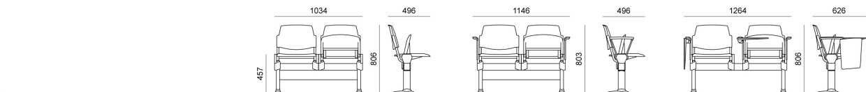
PANCA RIBALTABILE | TIP-UP BENCH
