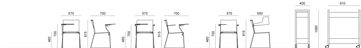
SEDIA CON SCRITTOIO + CARRELLO PORTA TAVOLETTE | CHAIR WITH REMOVABLE WRITING TABLE + TROLLEY FOR WRITING TABLES
