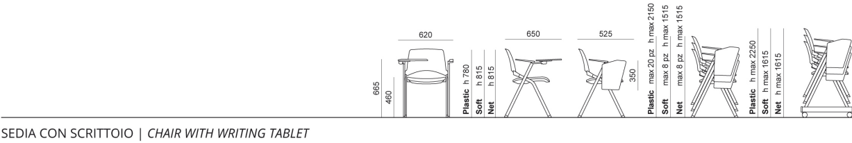
SEDIA CON SCRITTOIO | CHAIR WITH WRITING TABLET
