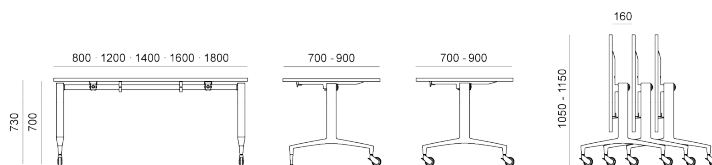
TAVOLO RIBALTABILE CON RUOTE E PIEDINI COMPENSATORI | FLIP TOP TABLE WITH CASTORS AND ADJUSTABLE GLIDES
