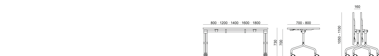
TAVOLO RIBALTABILE SU RUOTE | FLIP TOP TABLE ON CASTORS
